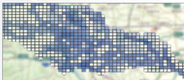
数値モデルによる有害化学物質の環境中濃度の推計事例 上: METI-LISによる大気中濃度分布の推計 下: AIST-SHANELによる河川での水質濃度分布の推計
