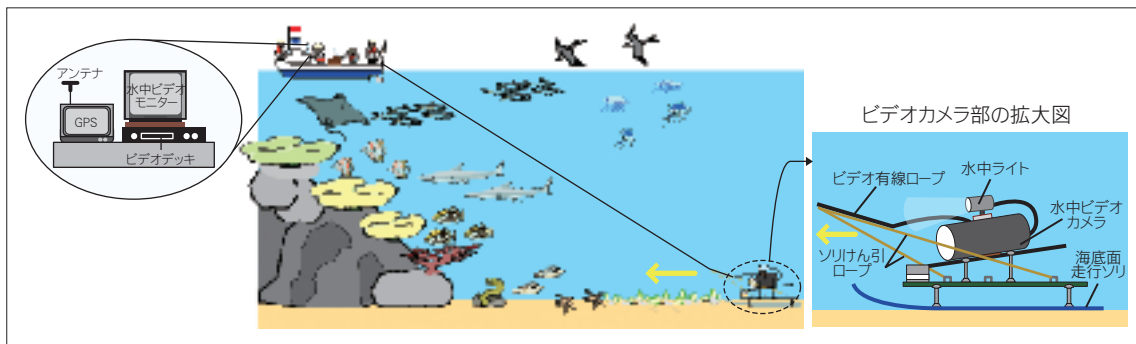
図1 水中ビデオによる曳航撮影システムの概要
