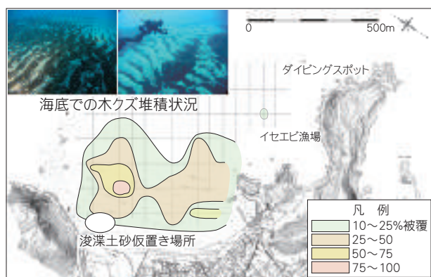
図2 木クズの堆積分布図(図中の写真は堆積・被覆した木クズ)
