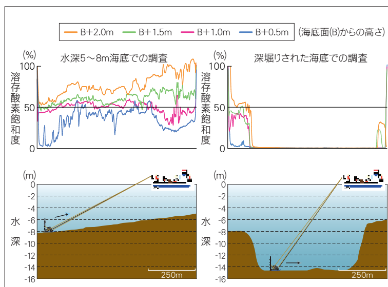
図4 深堀りされた海底(右)で観測した貧酸素水の発生状況
