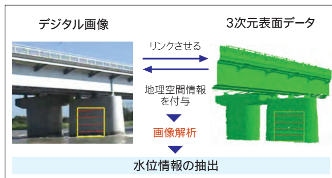
3次元データを使用した水位の自動計測処理のイメージ
