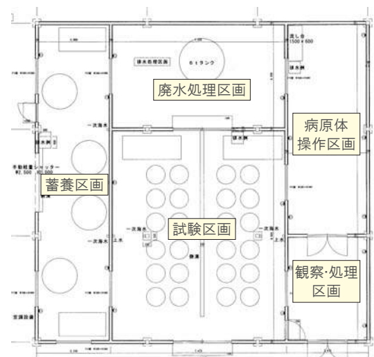
図1 閉鎖系飼育試験施設平面図
