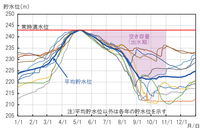
図2 農業用ダムの貯水位の年間変動例
